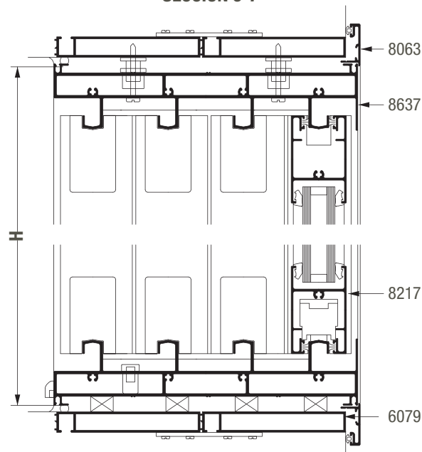
SECCION 6-7
