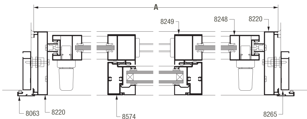
SECCION 11-12-13-14
