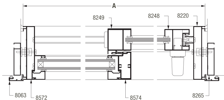
SECCION 1-2-3
