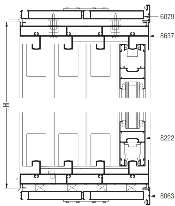
SECCION 13-14
